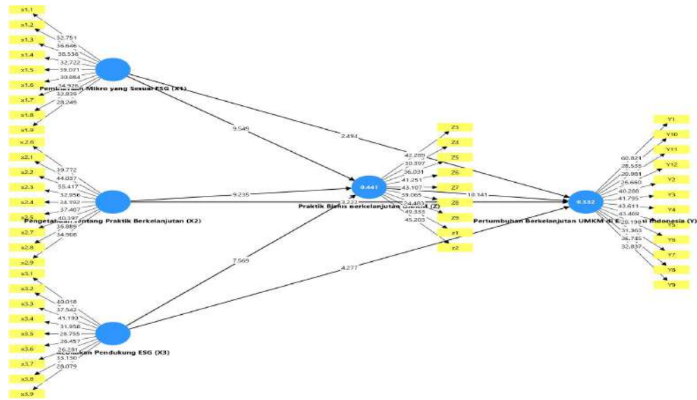
Gambar 1. Model Struktural (Hasil PLS-SEM)
